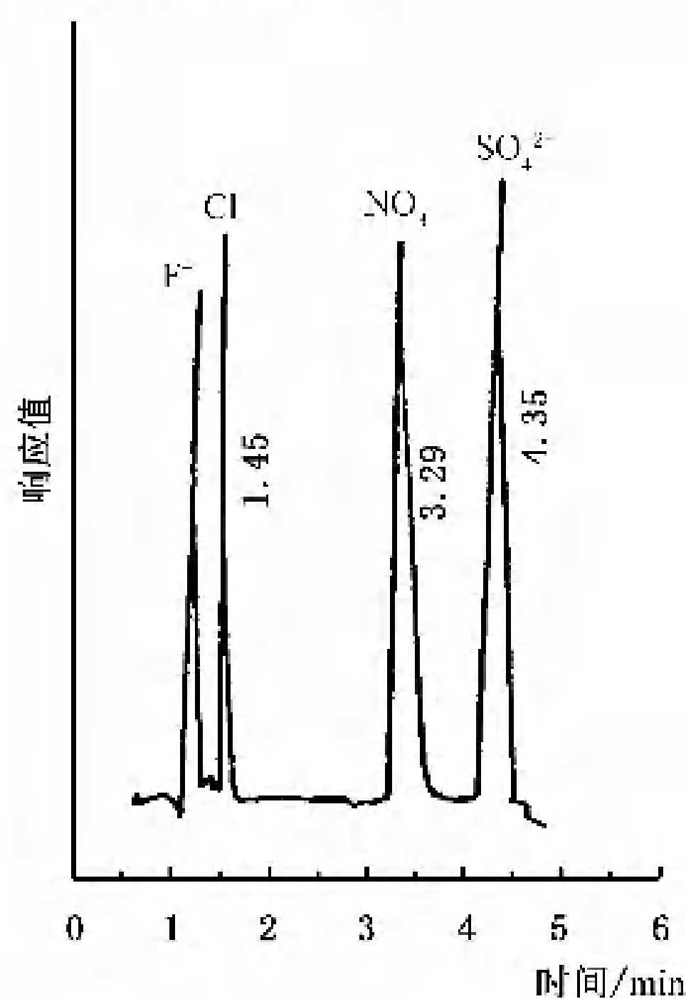
图 1 离子色谱图
